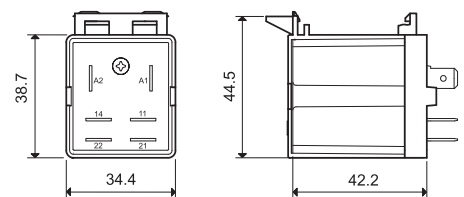
065.08 con relé
