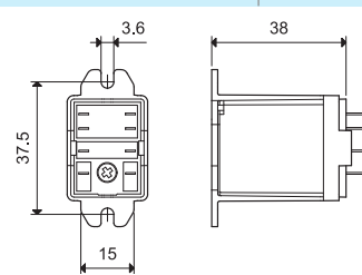
056.25 con relé
