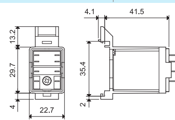
056.27 con relé
