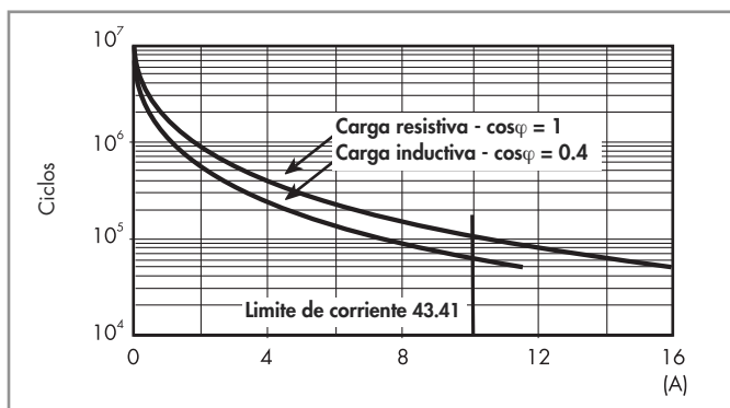
F 43 - Vida útil eléctrica (AC) en función de la carga
