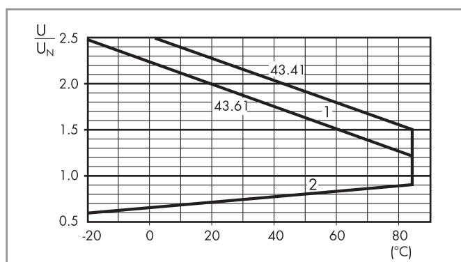
R 43 - Campo de funcionamiento de la bobina DC en función de la temperatura ambiente
