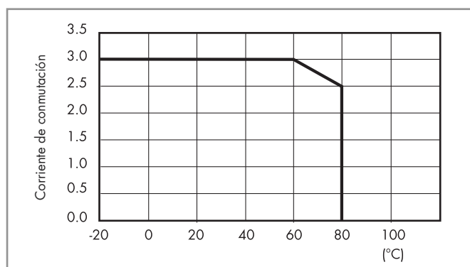
L 41 - Corriente de conmutación en función de la temperatura ambiente Salida 3 A AC
