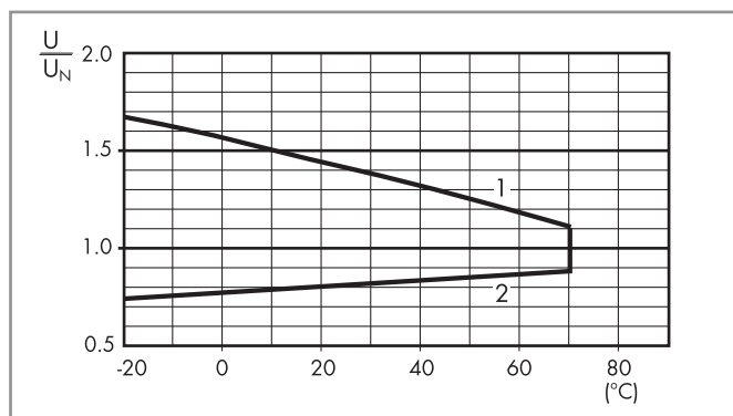
R 41 - Campo de funcionamiento de la bobina AC en función de la temperatura ambiente
