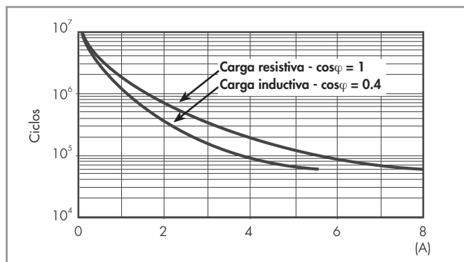
F 41 - Vida útil eléctrica (AC) en función de la carga Tipo 41.52
